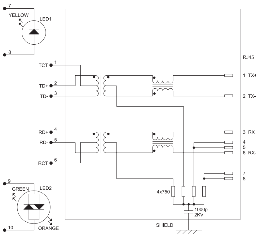
Rysunek 3. Schemat wewnętrzny gniazdka Ethernet
