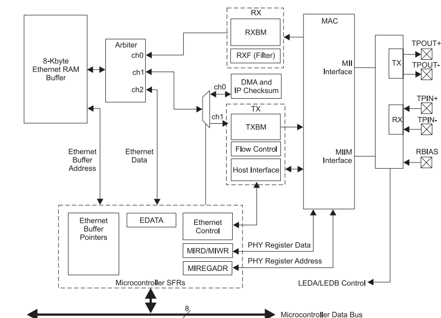
Rysunek 2. Schemat blokowy kontrolera Ethernet układu PIC18F67J60
