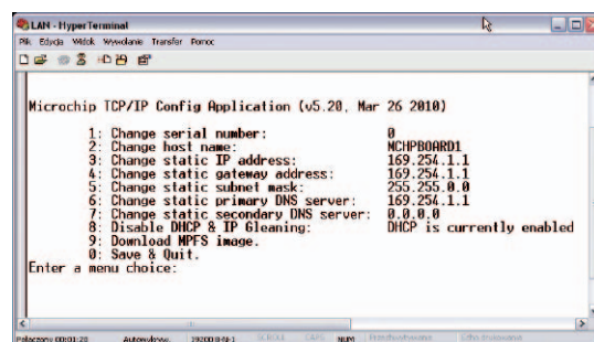
Rysunek 7. Menu główne służące do nastaw parametrów
