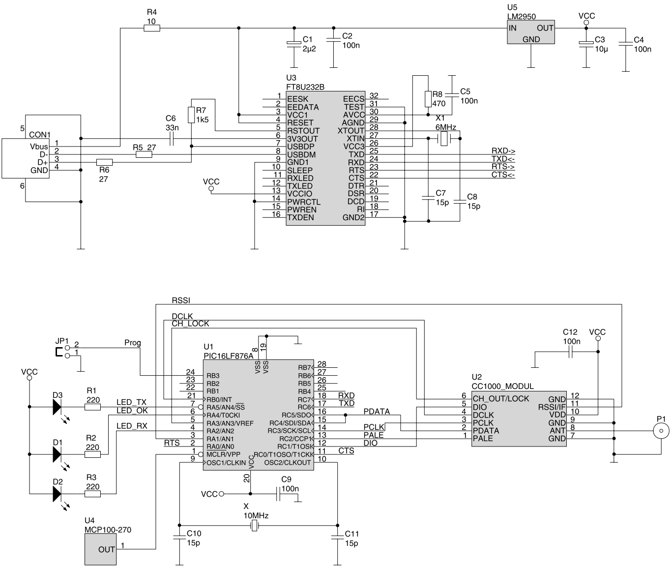
Rys. 2. Schemat elektryczny modemu
