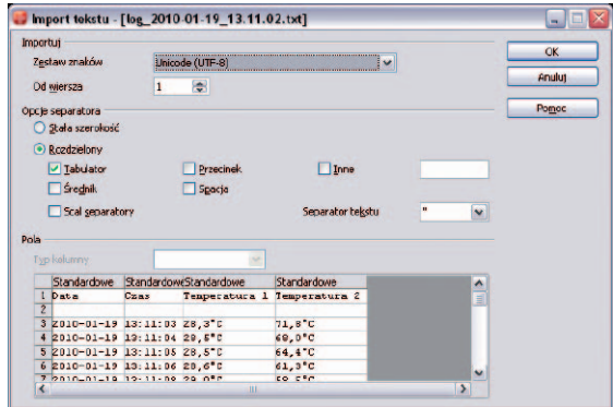
Rys. 4. Okno konfiguracyjne importu danych z pliku
